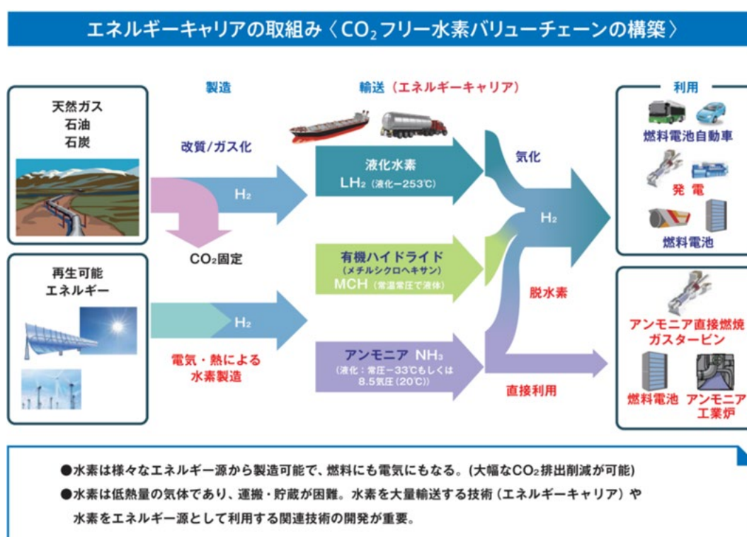
図 4 水素サプライチェーンのイメージ図 (IAE: CO 2 フリー水素普及シナリオ研究会)
