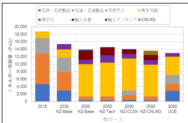
図4. 2030年の基準ケースおよび2050年の各ケースにおける日本の一次エネルギー供給
